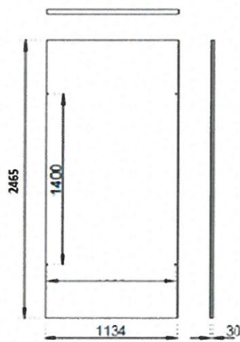
Figura 4. Desen indicativ - Detalii panouri fotovoltaice – conform specificațiilor din prezentul caiet de sarcini – dimensiunile de referință sunt 2465 x 1134 x 30 mm ( \pm 5 mm)
