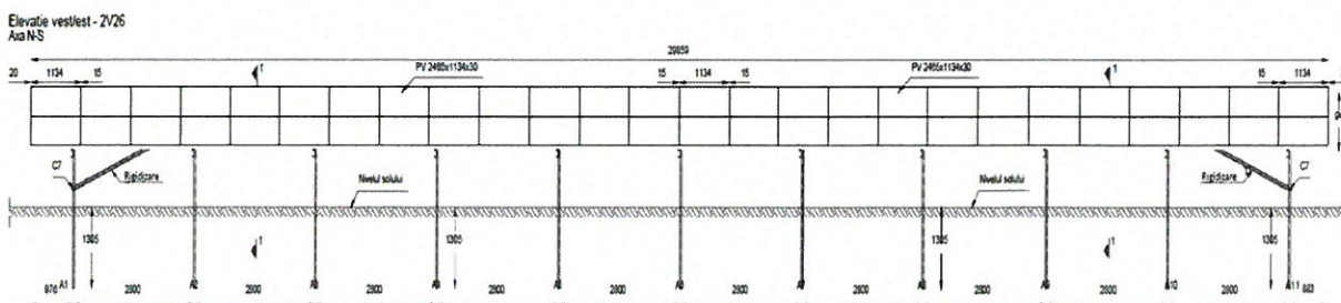
Figura 2. Desen indicativ - Detalii structură – vedere structură (Est – Vest)
