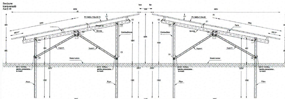
Figura 1. Desen indicativ - Detalii structură – secțiune transversală
