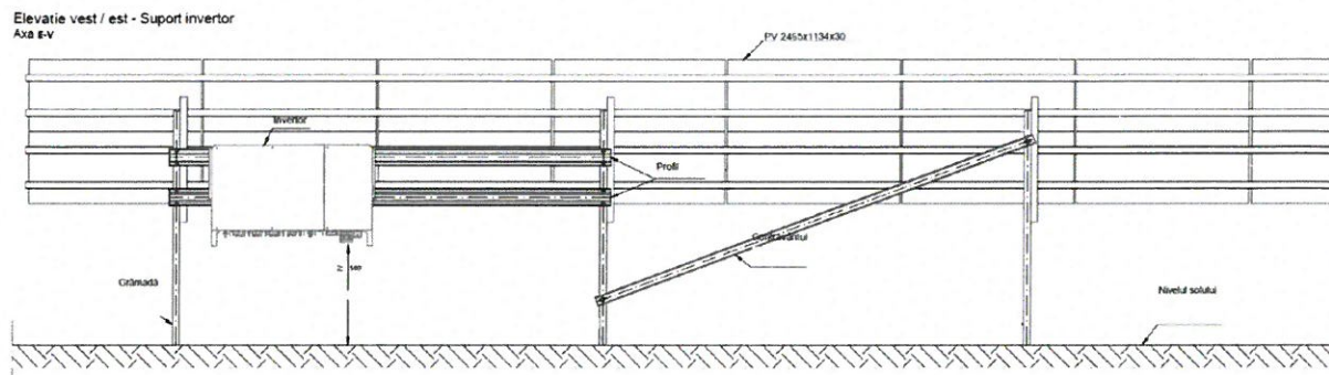
Figura 3. Desen indicativ – Detalii structura – soluție pentru structura de montare a invertoarelor
